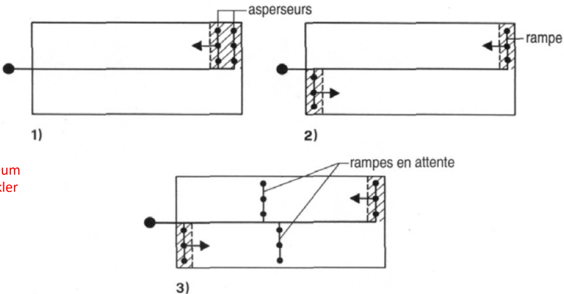
Fig. 27 : Schéma de principe d'installations en couverture partielle
